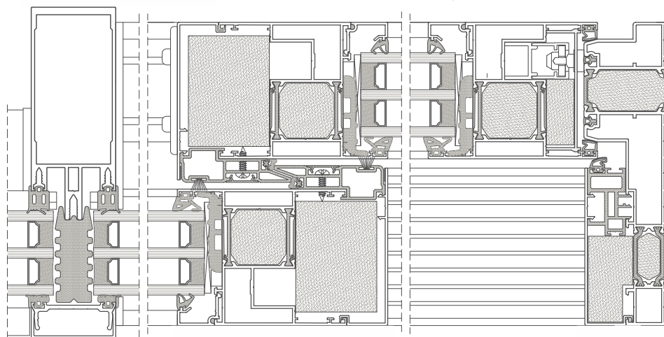
PRŮŘEZ DVEŘMI DP180 PRIMEVIEW Š FASÁDOU
