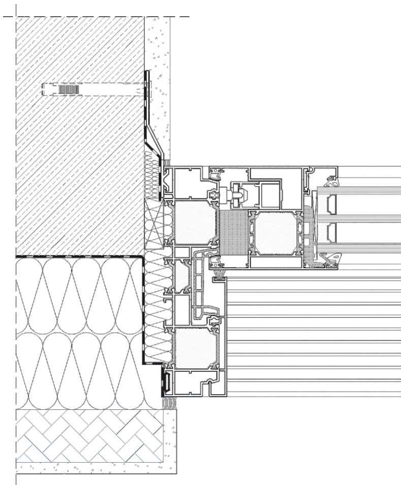
DP 180 PRIMEVIEW - BOČNÍ ČÁST
