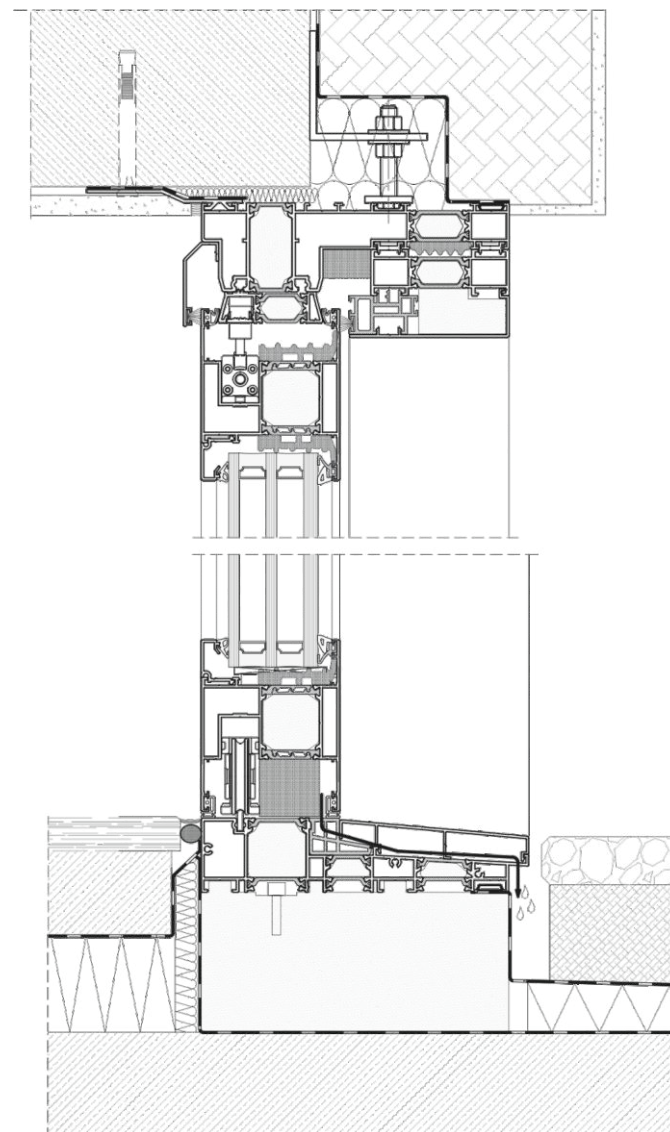
PRŮŘEZ DP 180 PRIMEVIEW NÍZKÝ PRÁH - POSUVNÉ KŘÍDLO.
