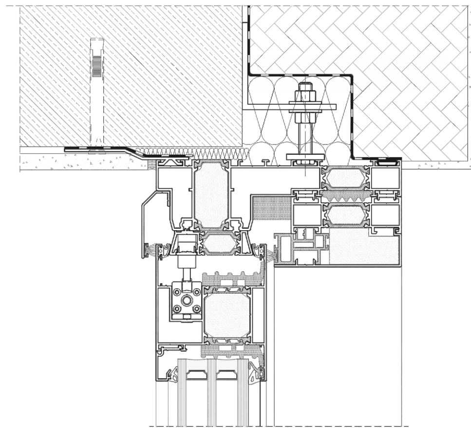
DP 180 PRIMEVIEW HORNÍ ČÁST
