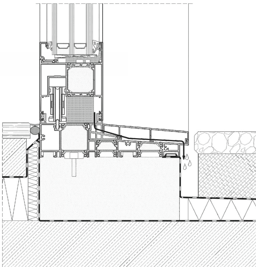
DP 180 PRIMEVIEW DOLNÍ ČÁST
