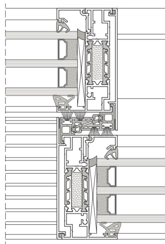
PRŮŘEZ SLOUPKEM DP 180 PRIMEVIEW
