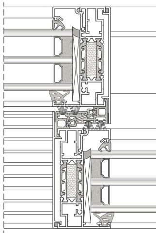
PJŪVIS PER DP 180 PRIMEVIEW SIAURĄ STATRAMSTĮ
