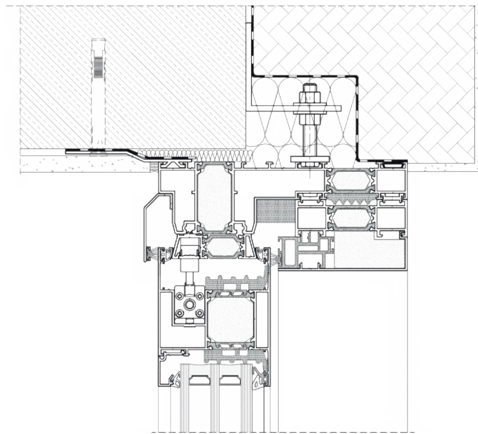
PJŪVIS PER DP 180 DURIS FASADE
