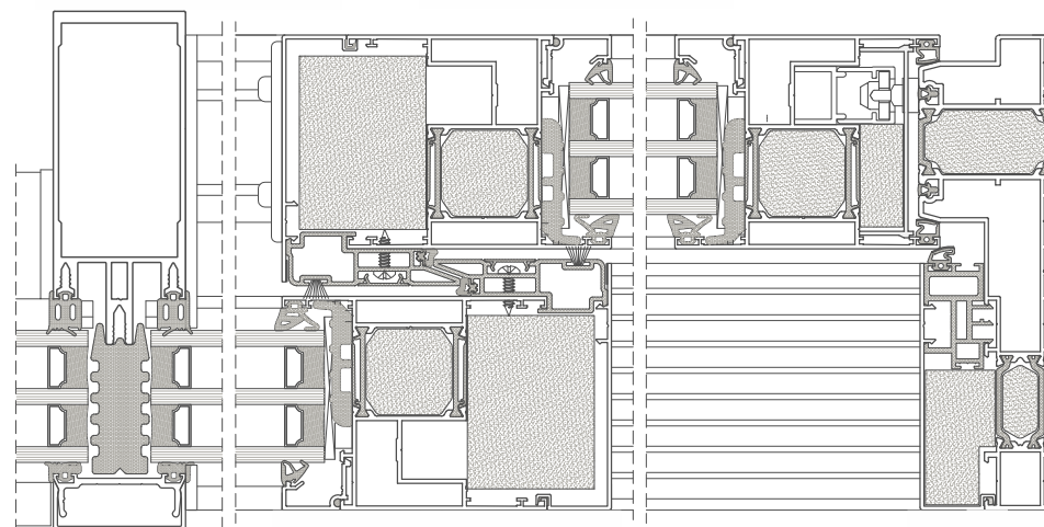
PJŪVIS PER DP 180 PRIMEVIEW DURIS SU FASADU
