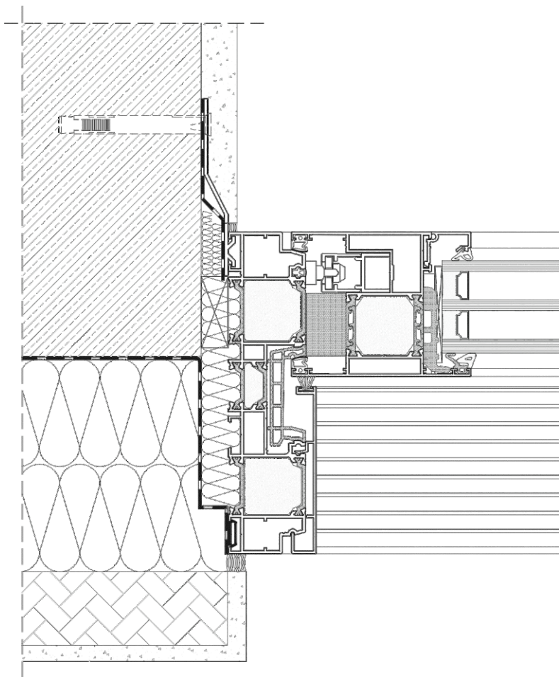
DP 180 PRIMEVIEW – ŠONINIS PJŪVIS
