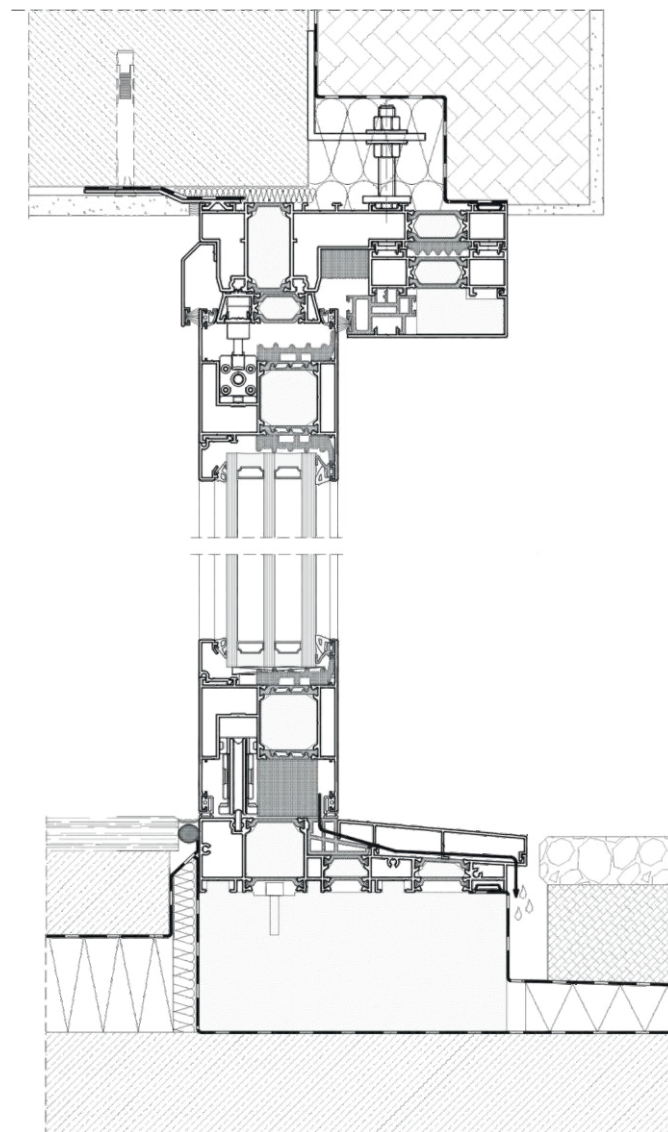
DP 180 ŽEMAS SLENKSTIS – STUMDOMA VARČIA
