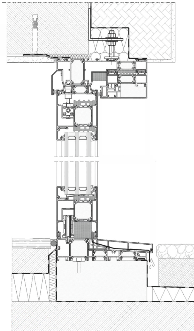
DP 180 PRIMEVIEW ŽEMAS SLENKSTIS – STUMDOMA VARČIA
