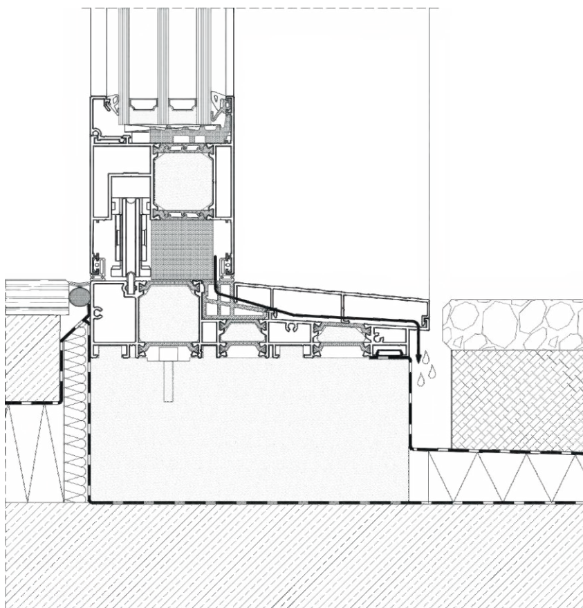
PJŪVIS PER DP 180 GLASS DURIS
