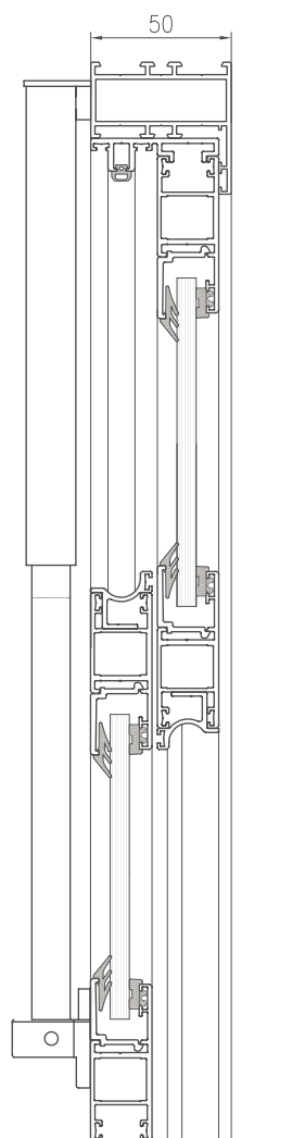
UŽDARYTO APTARNAVIMO LANGELIO PBI 50N PJŪVIS
