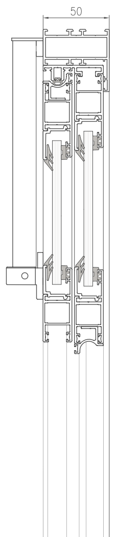
ATIDARYTO APTARNAVIMO LANGELIO PBI 50N PJŪVIS
