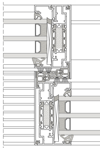
PRZĘKÓJ PRZĘZ WĄSKI SŁUPEK DP 180 PRIMEVIEW
