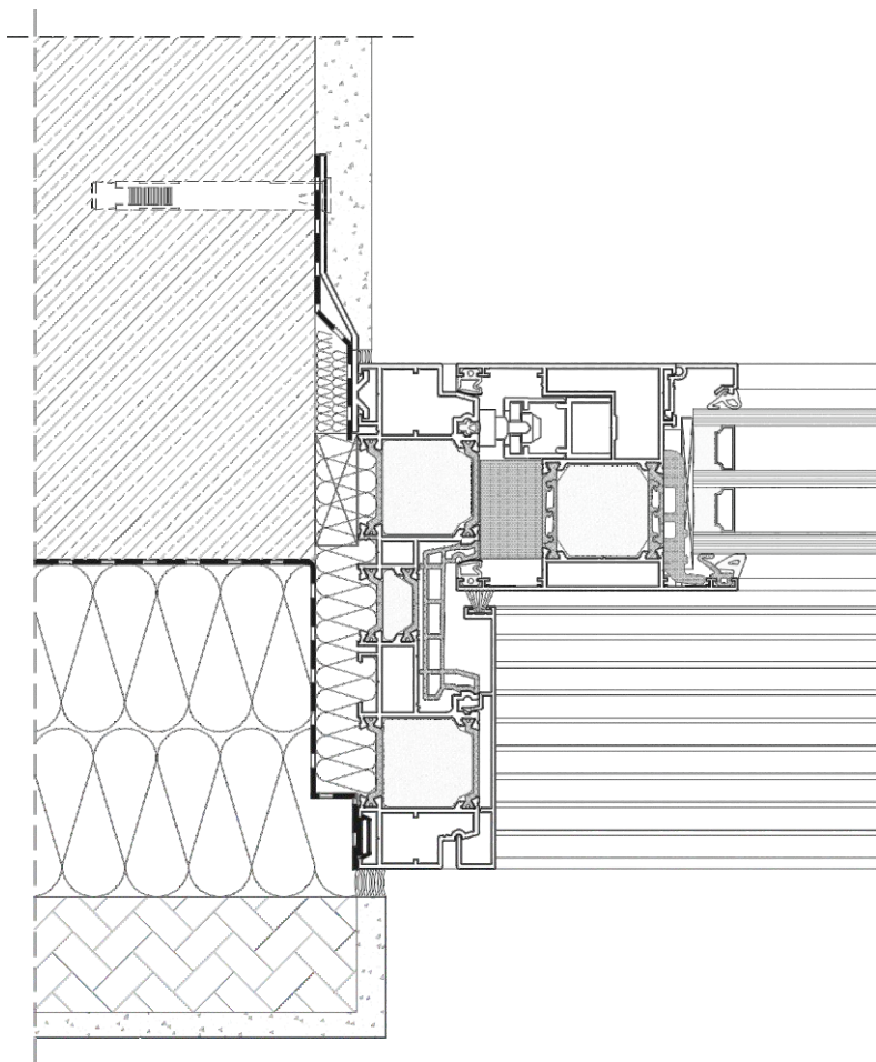
DP 180 PRIMEVIEW – PRZĘKÓJ BOCZNY
