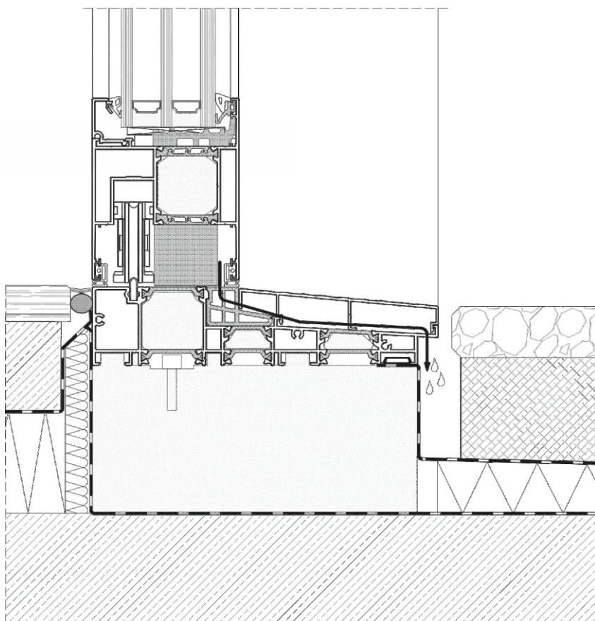
DP 180 PRIMEVIEW - SPODNÁ SEKCIA
