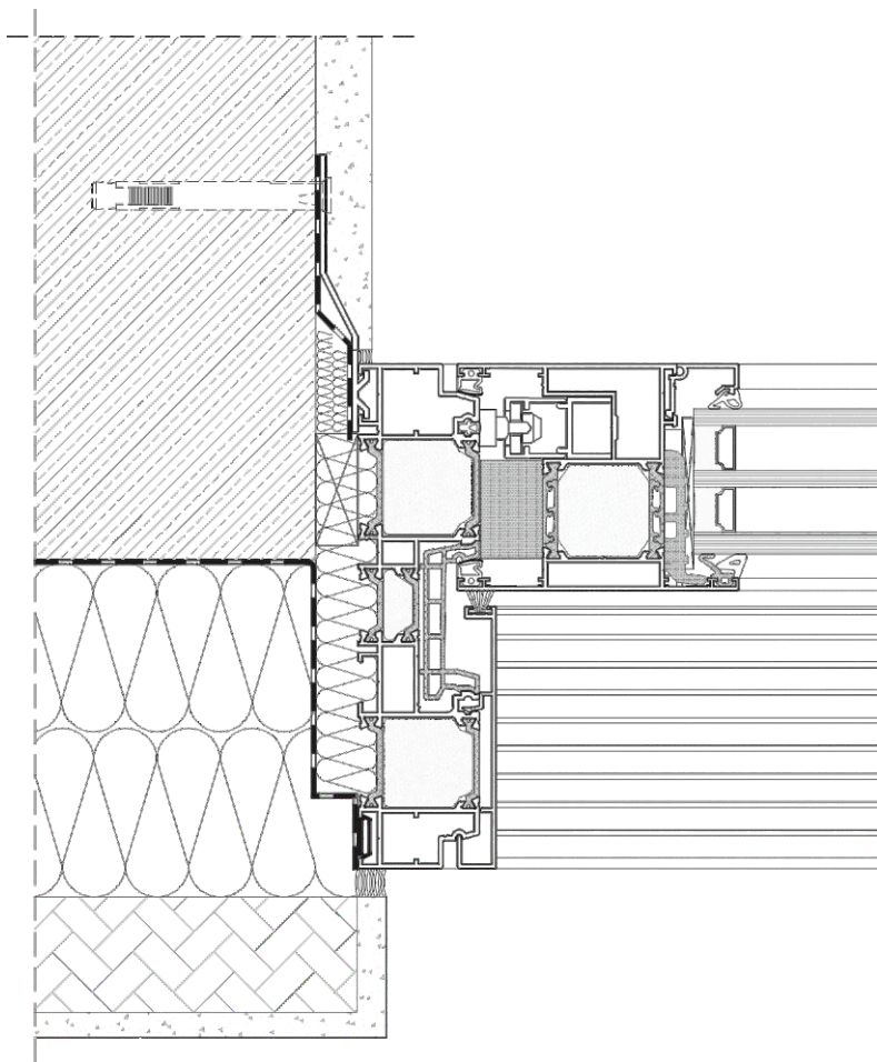
DP 180 PRIMEVIEW - BOČNÁ ČASŤ
