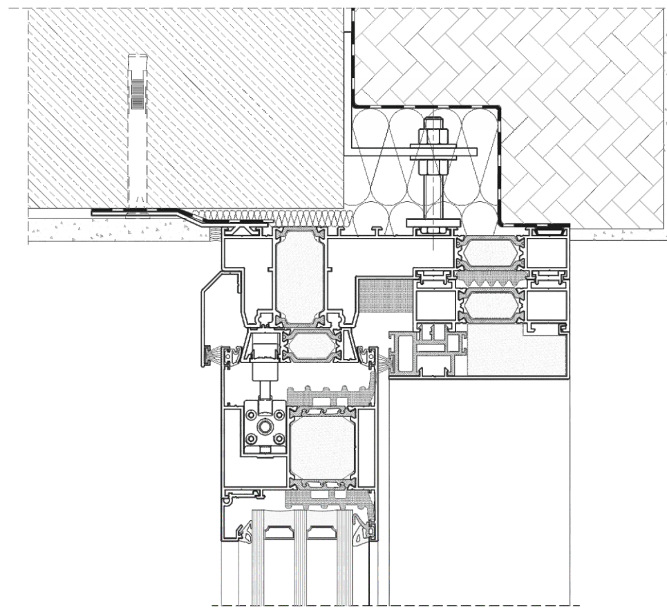
DP 180 PRIMEVIEW - HORNÁ ČASŤ
