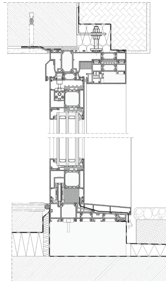
PRIEREZ DP 180 PRIMEVIEW NÍZKY PRAH - POSUVNÉ KRÍDLO
