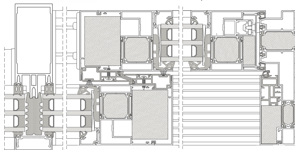
PRIEREZ DVERAMI DP 180 PRIMEVIEW S FASÁDOU
