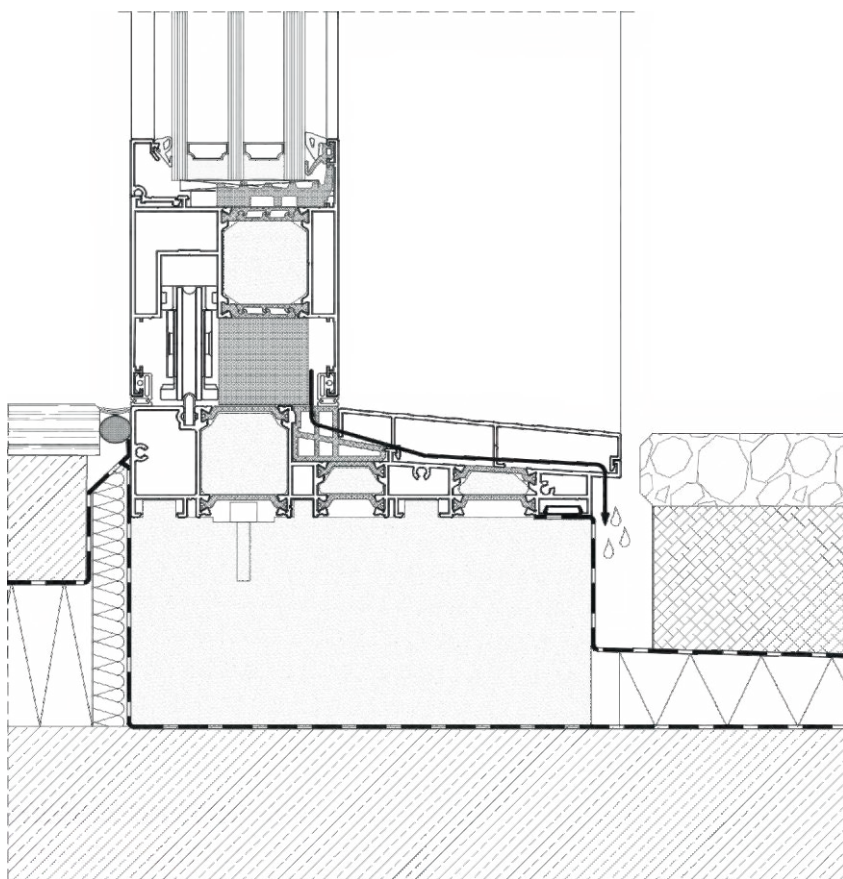
DP 180 - SPODNÁ SEKCIA
