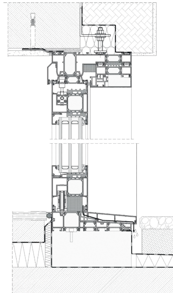
PRIEREZ DP 180 NÍZKY PRAH - POSUVNÉ KRÍDLO
