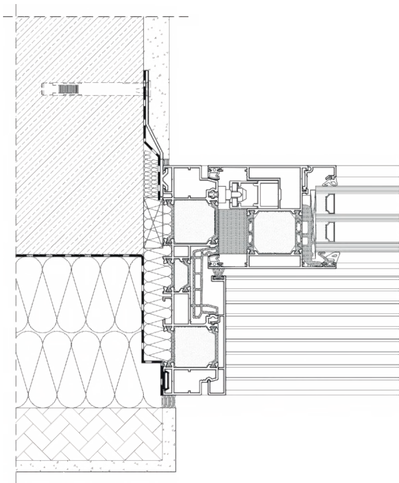
DP 180 - BOČNÁ ČASŤ
