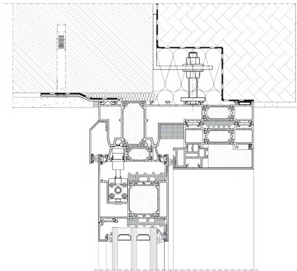
DP 180 - HORNÁ ČASŤ
