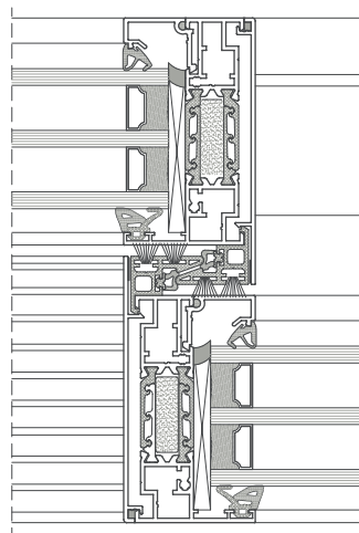
PRIEREZ STĽPIKOM DP 180
